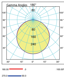
Işık Şiddeti Dağılım Eğrisi
