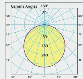
Işık Şiddeti Dağılım Eğrisi Light Distribution Curve
